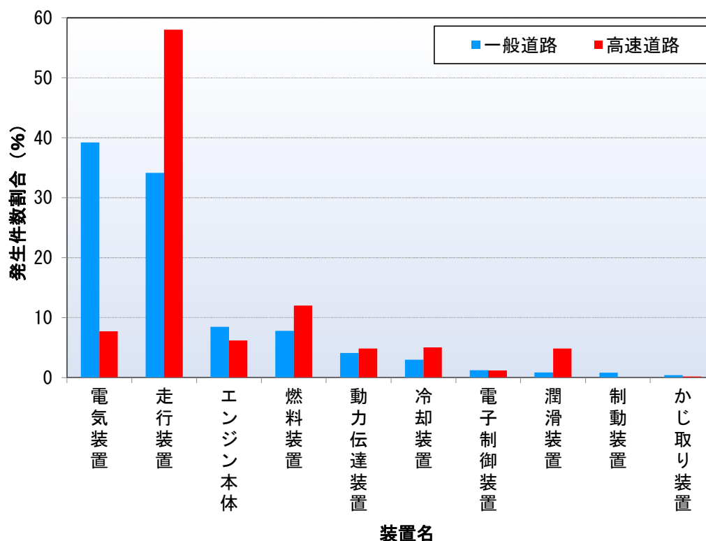
図1 道路別装置別故障発生件数の割合
