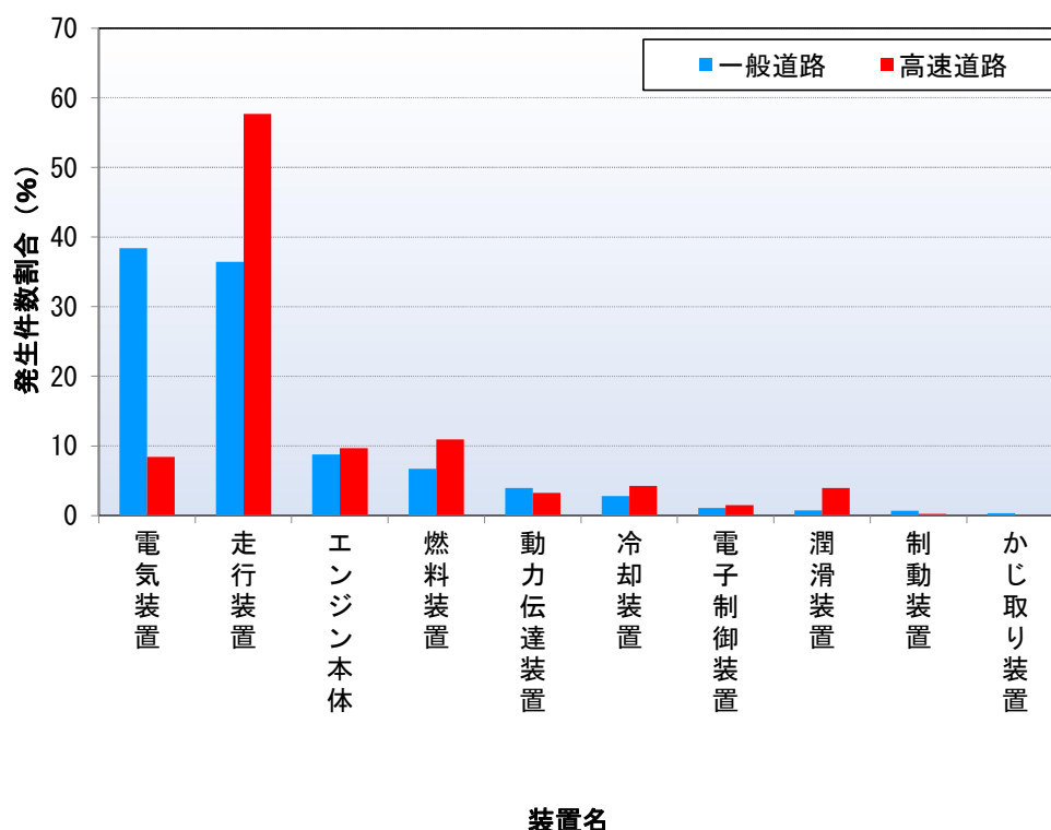
図1 道路別装置別故障発生件数の割合
