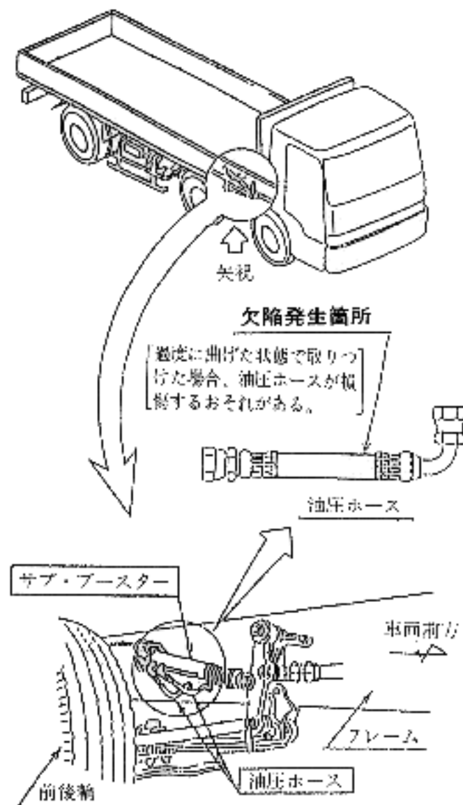
矢視図
