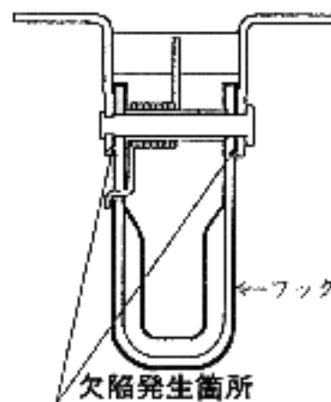
矢視A 止め金具断面
