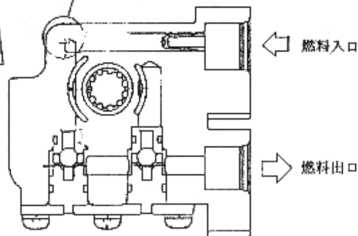
[高圧燃料ポンプ内燃料通路断面図]
