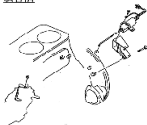
燃料カット装置(電磁石式)
