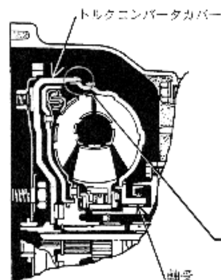
断面図
