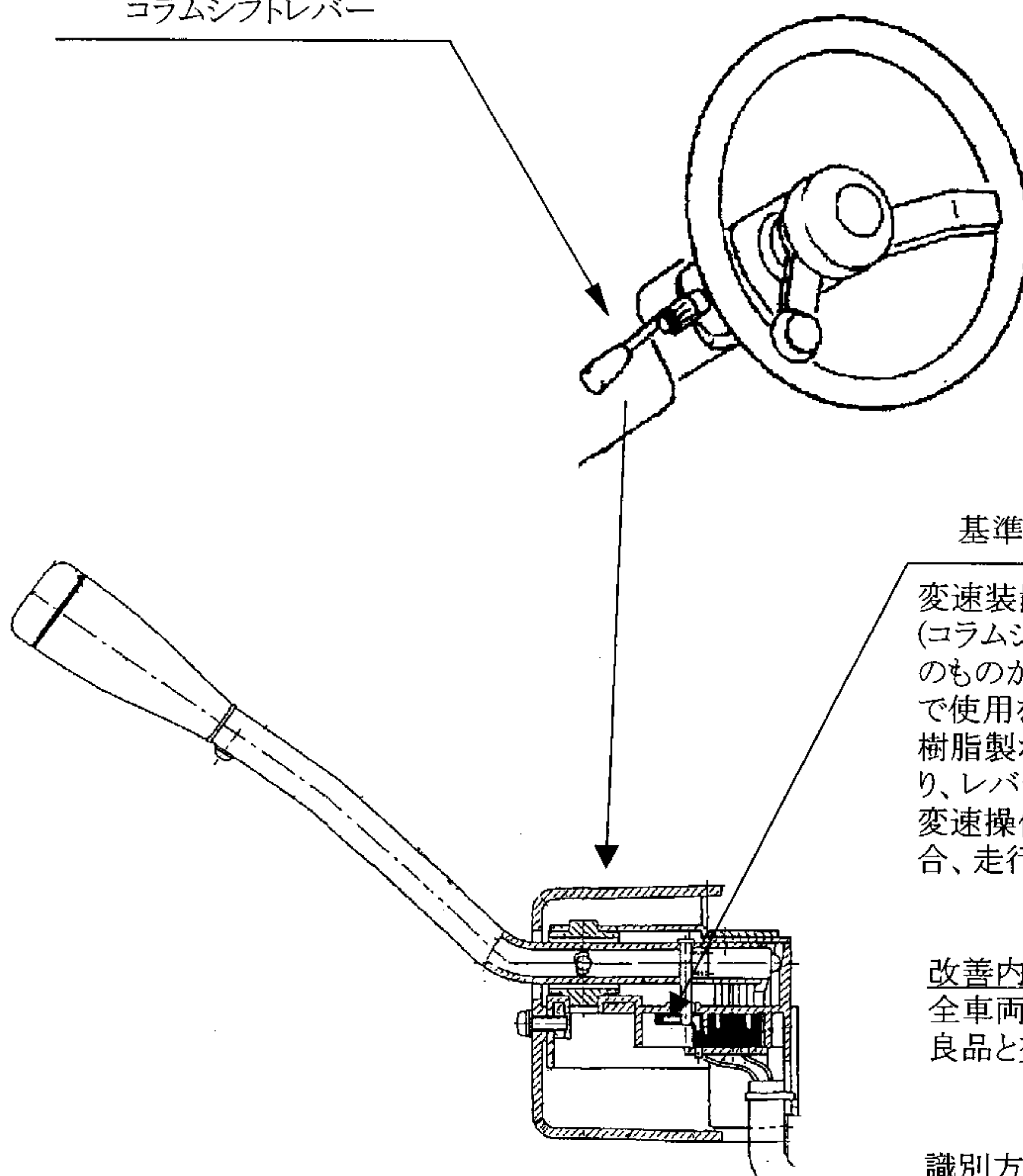
コラムシフトレバー断面図
