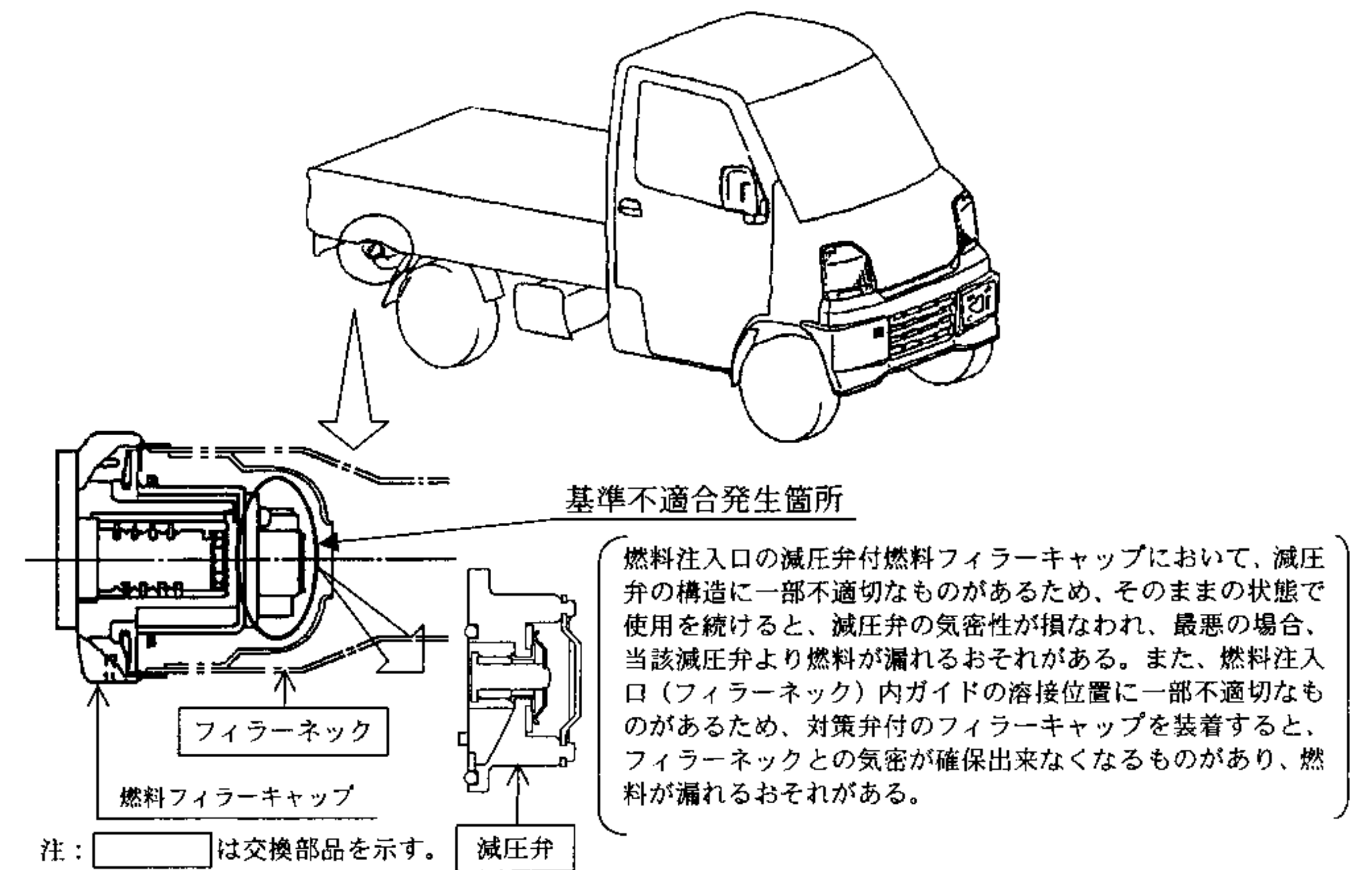
改善箇所説明図（フィルターキャップ）
