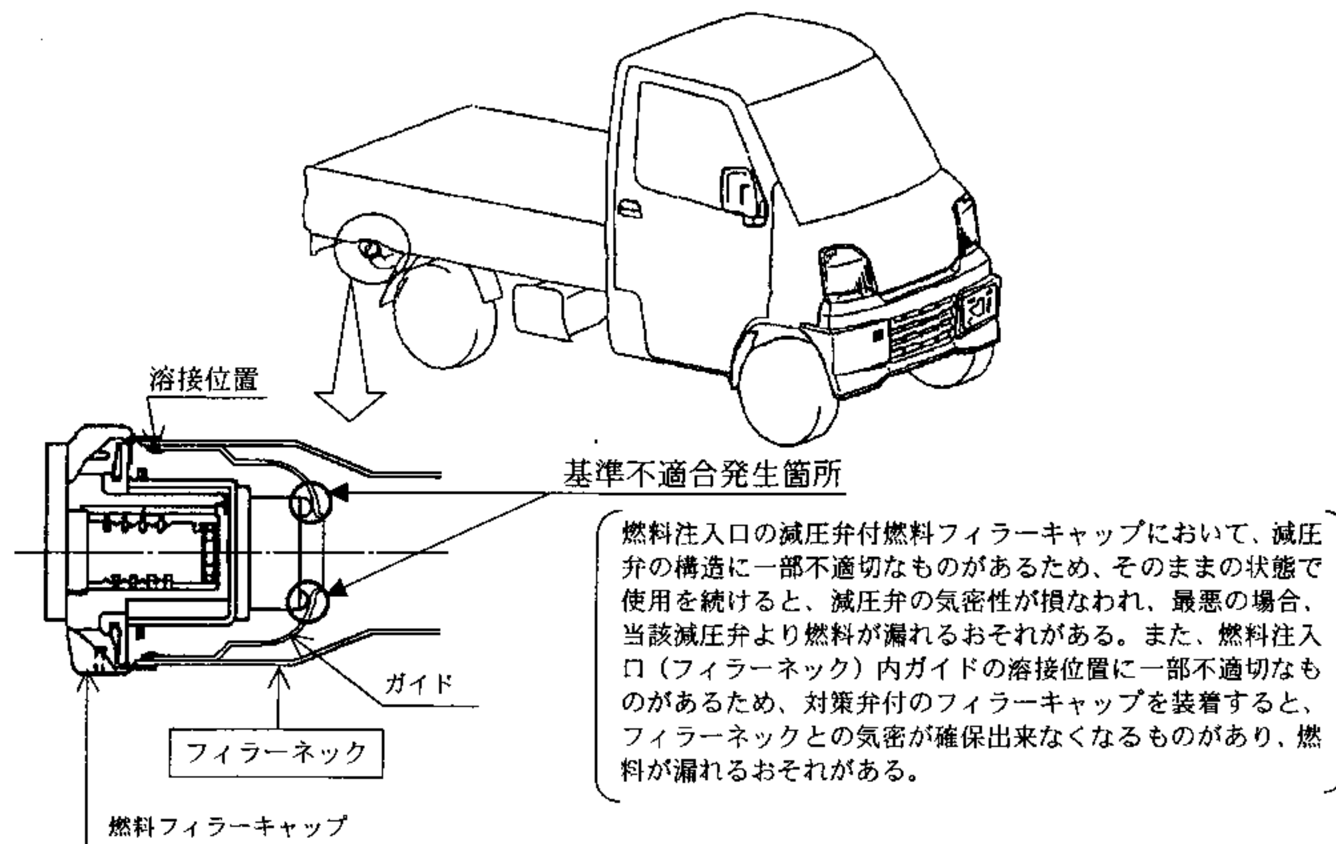
改善箇所説明図（フィルターネック）
