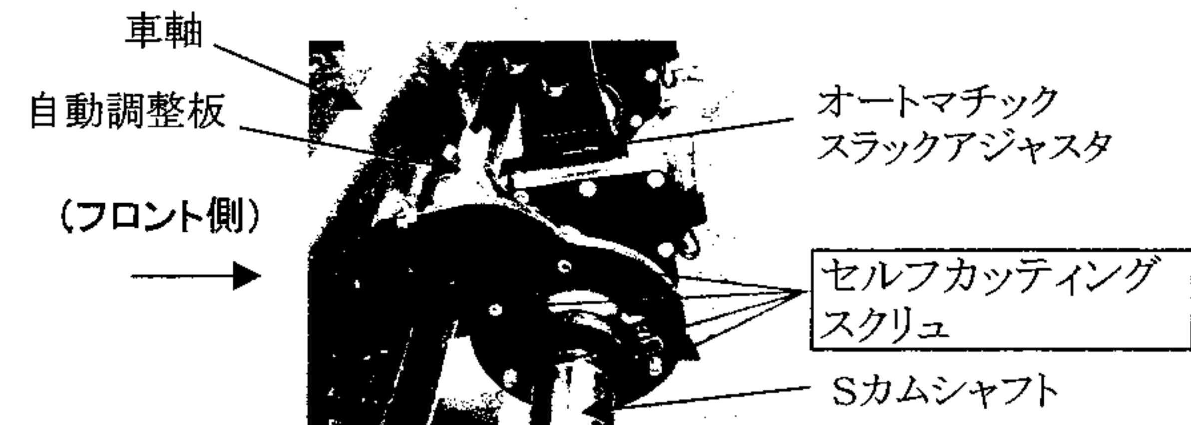
(Sカムシャフト、オートマチックスラックアジャスタの固定部)
