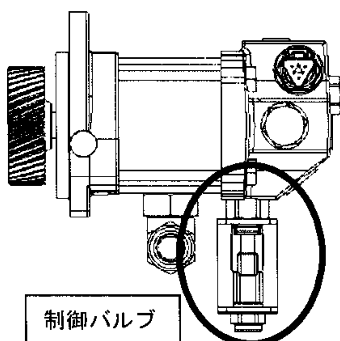
ブレーキ用油圧ポンプ
