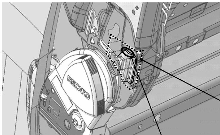
基準不適合発生箇所（突起部）
