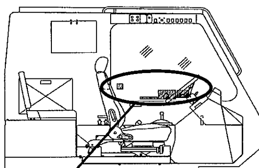
運転者席断面図（左内側を示す）
