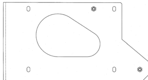
ブラケットB強度アップ品 形状変更 および 板厚増加 6mm⇒9mm
