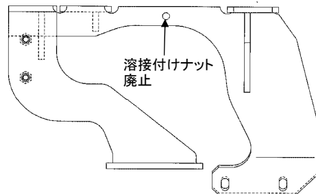
ブラケットA強度アップ品 形状変更 および 板厚増加6mm⇒9mm
