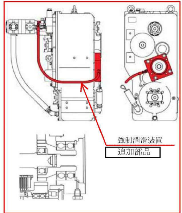
改善後構造(強制潤滑装置取付け)
