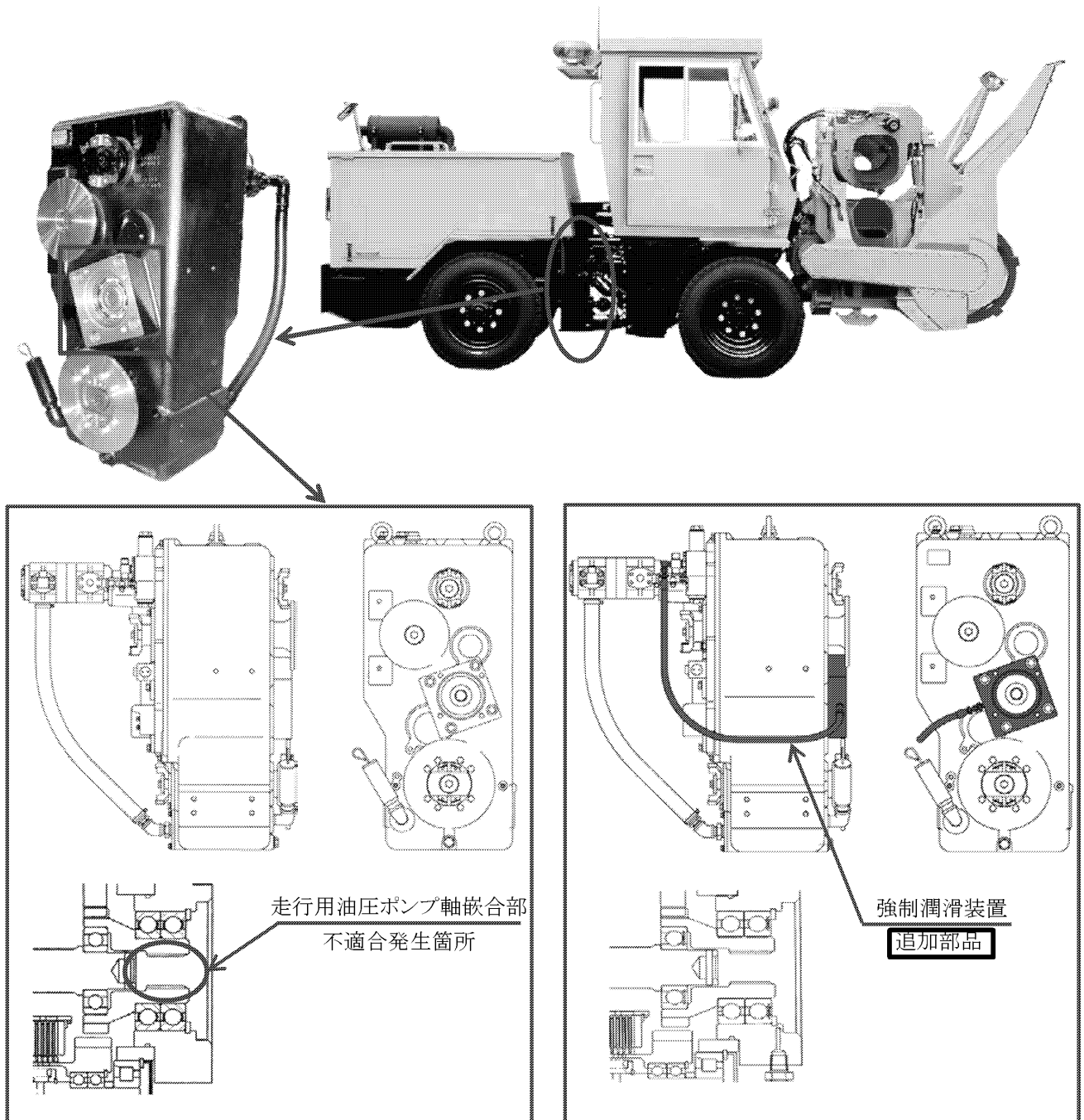
改善前構造
