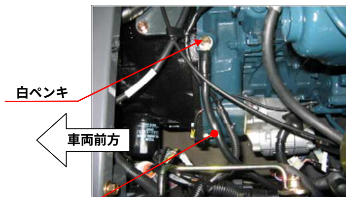
バッテリー～スタータモータ間の電気配線（一側）
