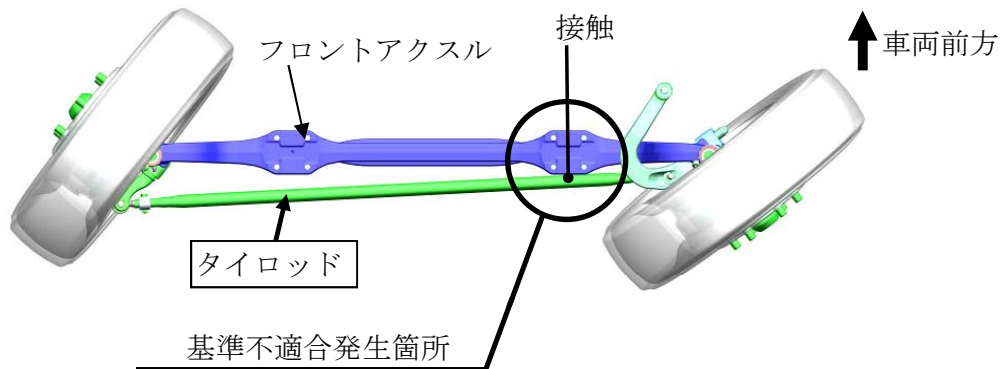
車両上方視
