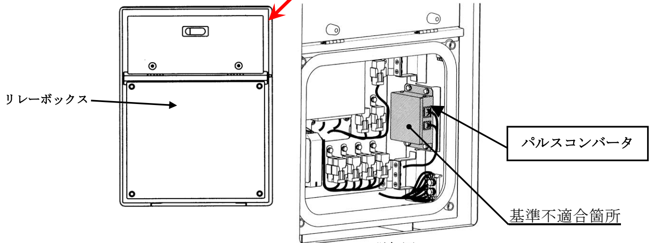
詳細図
