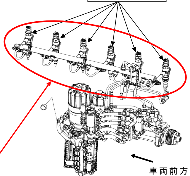
フューエルライン
