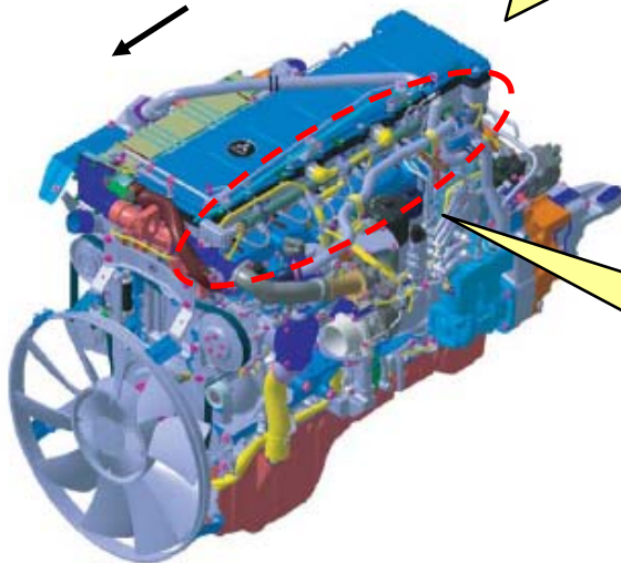
エンジン全体図
