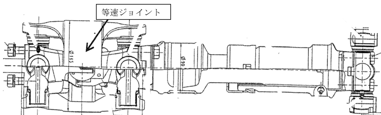
ニイガタ JDS-NR6A 外観側面図
