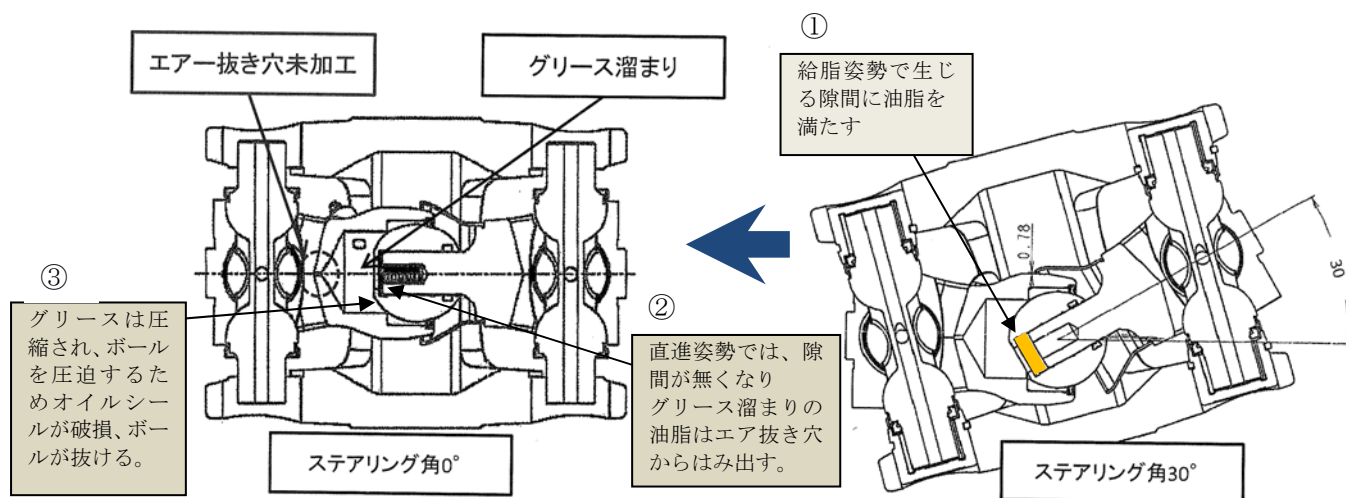
等速ジョイント断面図
