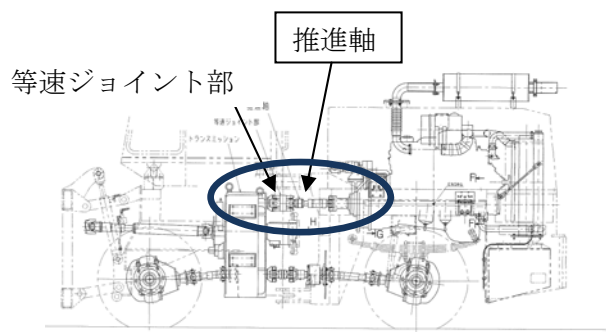
動力伝達図
