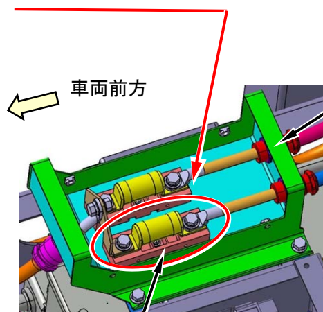
インバータB側ヒューズ
