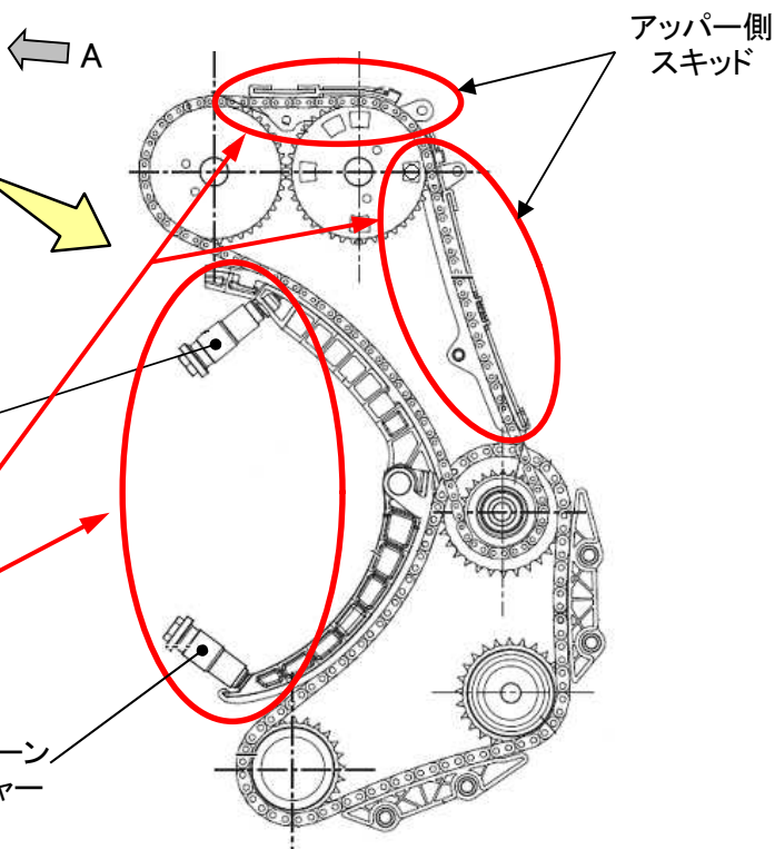
タイミングチェーンシステム (A 視)
