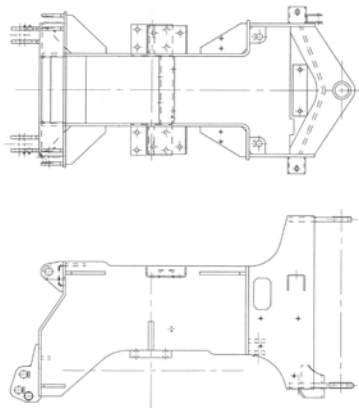
改造自動車 前フレーム
