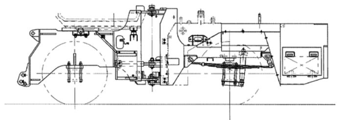
改造自動車 車枠
