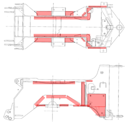
前フレームの補強箇所
