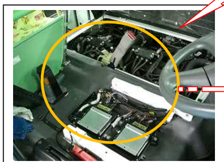
コントロールユニット及び E/ルーム間ハーネス交換
