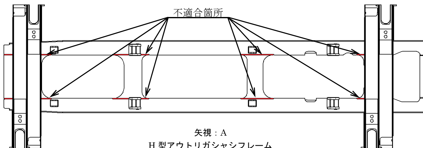
WDR-KRC013 (H型アウトリガ)
