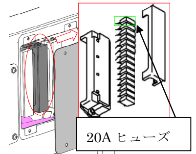
(E)運転席左側ランチボックスストレー内部
