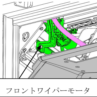
(A)正面上側（内装内部）
