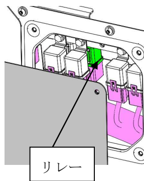
(C)運転席背面カバー内部
