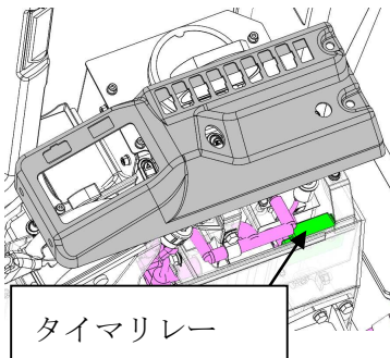
(B)運転席右側 コンソールカバー内部
