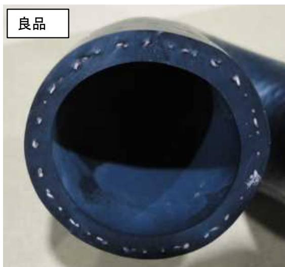
ラジエタホース (LOW側)
