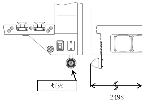
車両後面視
