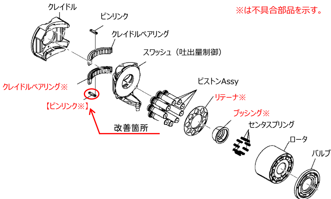
【ポンプ内部構成部品】
