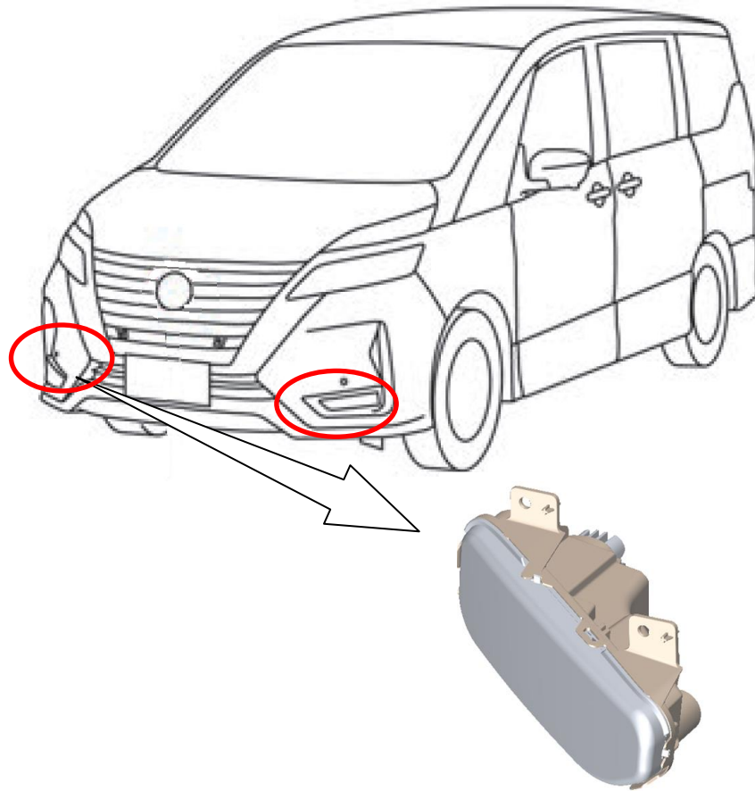
前部雾灯装置 (LED フォグランプ)
