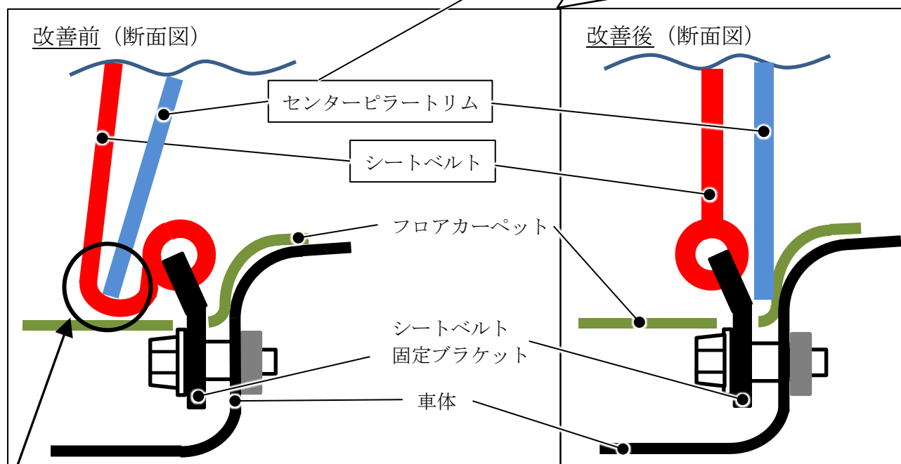
シートベルト 固定ブラケット
