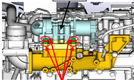
取付ボルト
