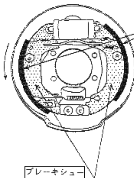
矢視断面図
