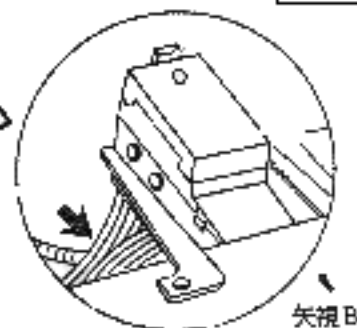
■対策箇所 その2 分電器
