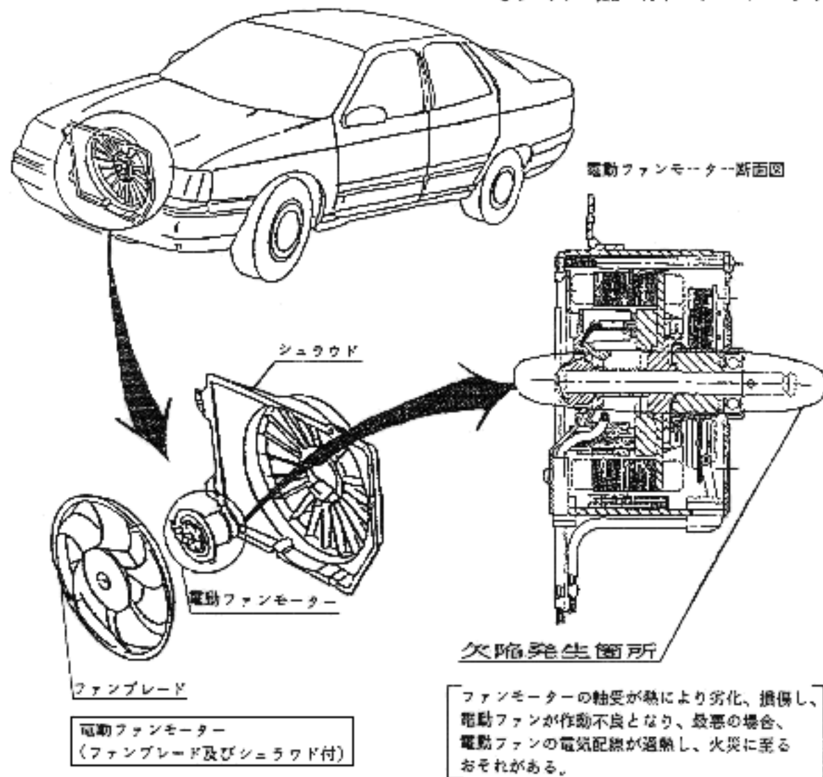
電動ファンモーター断面図
