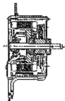
電動ファンモーター断面図
