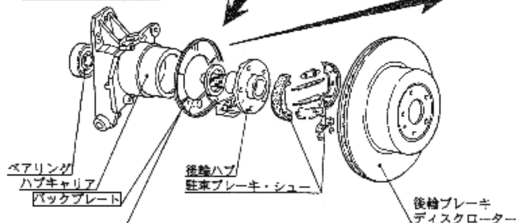
後輪駐車ブレーキ分解図
