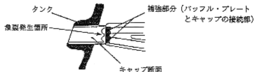
不具合箇所拡大断面図 (タンク上面からの図)
