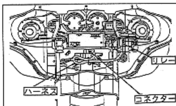
矢視 A フェアリツガカバーをはずした図
