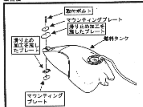
改善後
