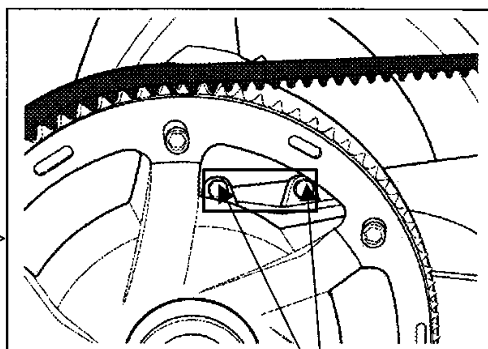
ブレーキキャリパ取付ボルト
