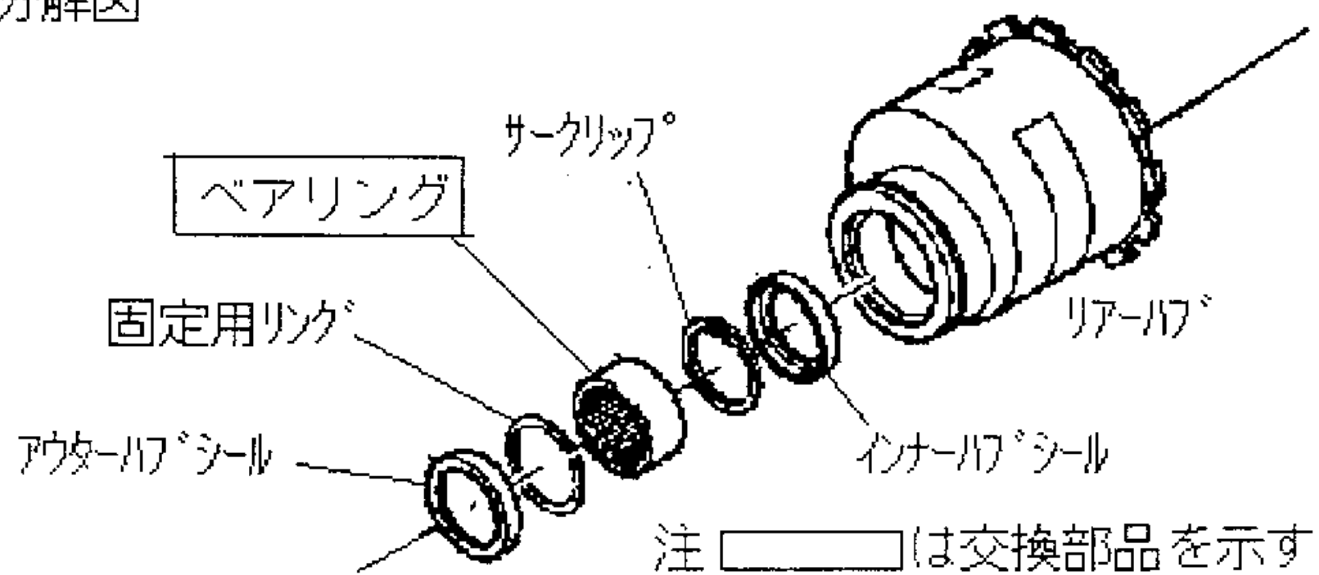
分解図
