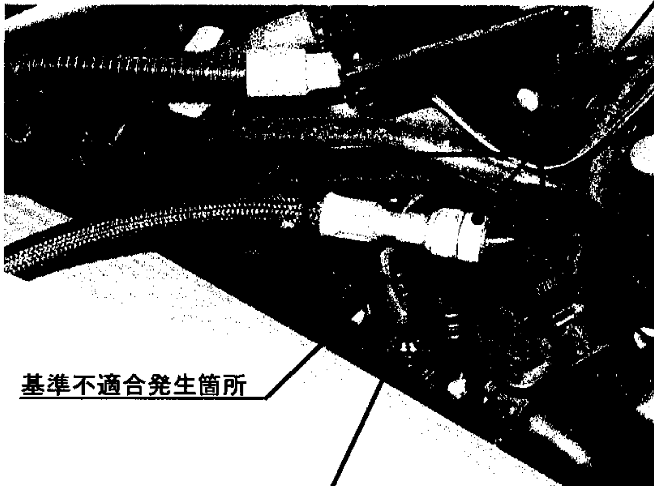
供給側燃料パイプ
