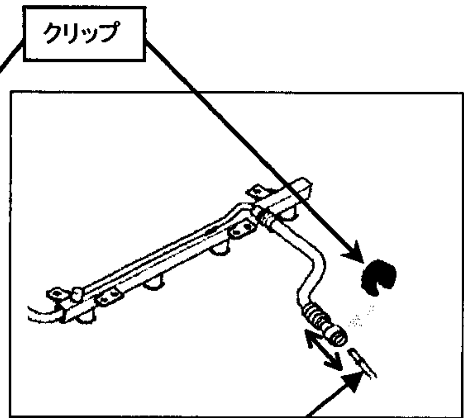
供給側燃料パイプ
