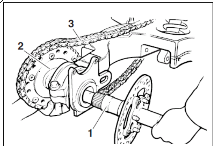
ブラケット取り付け図
