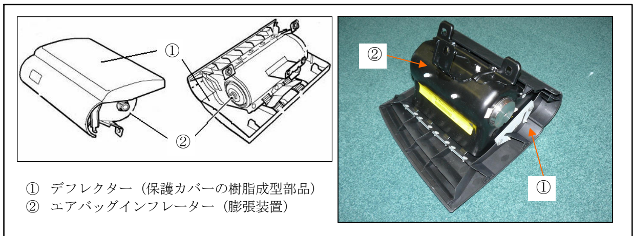
助手席エアバッグ装置
