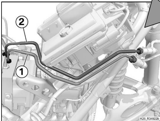
交換前の前輪用ブレーキ配管
