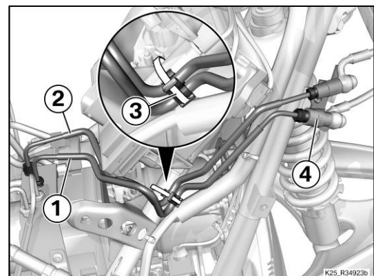
交換後の前輪用ブレーキ配管
