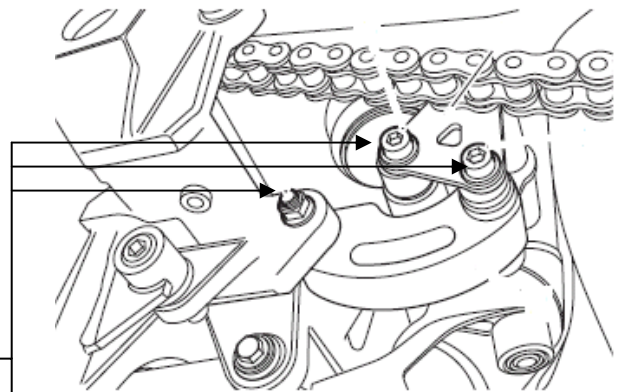
リヤサスペンションリンク部拡大図
