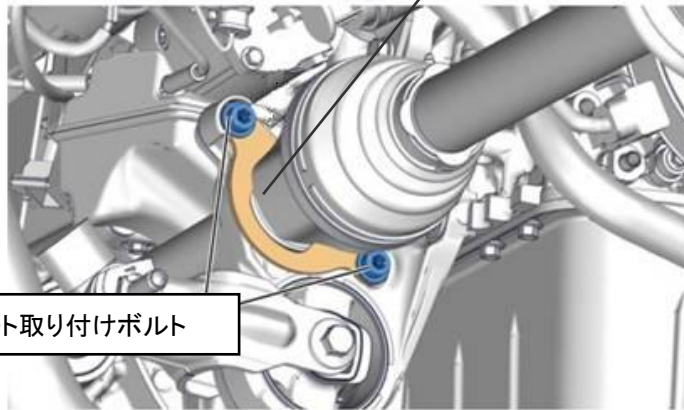
右側ドライブシャフトベアリングのリテーニングプレート
