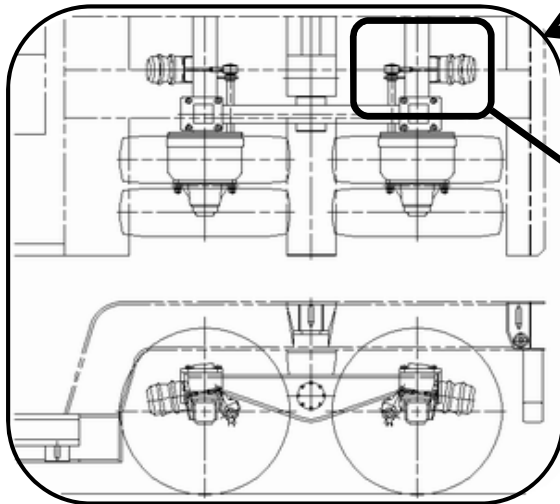
車軸詳細図
