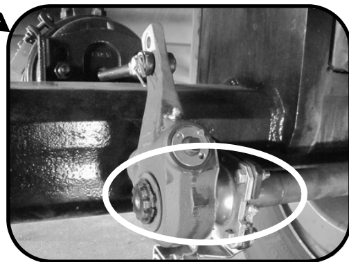
ブレーキカムシャフト スプライン部 (スラックアジャスター嵌合部)
