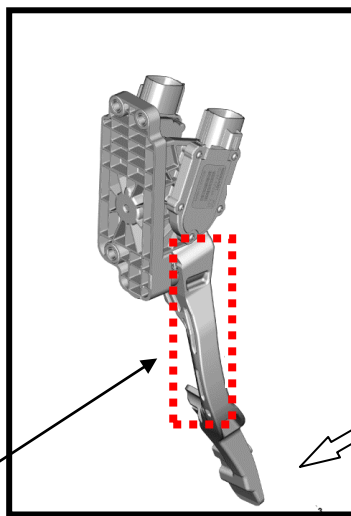
スロットルペダルアッセンブリー
